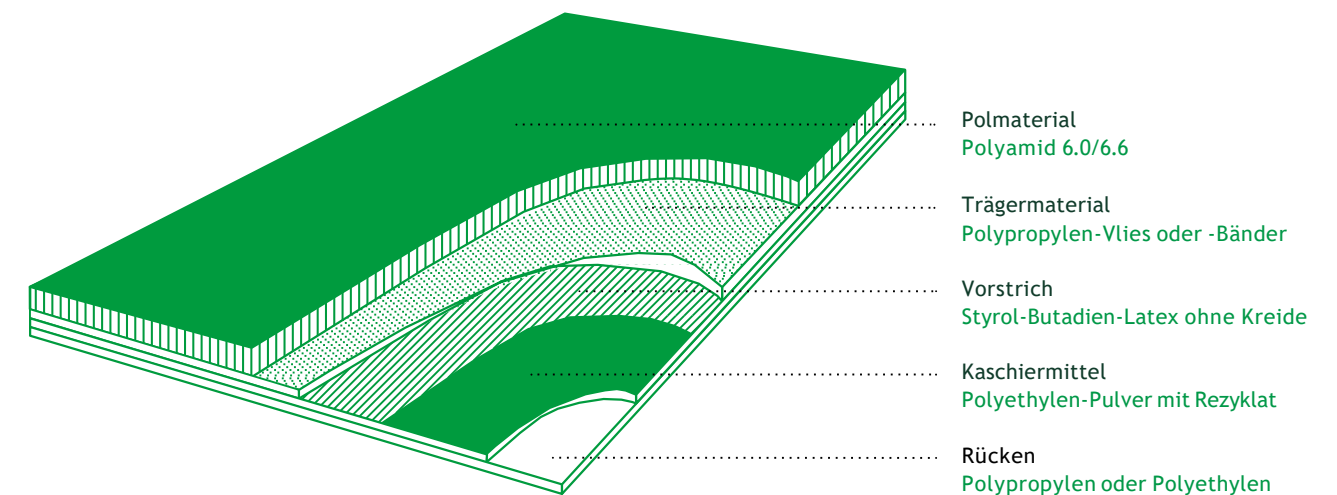
AUFBAU EINESTUFTEPPICHS
