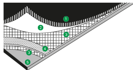
AUFBAU DER TEXTILES-RÜCKENBESCHICHTUNG
