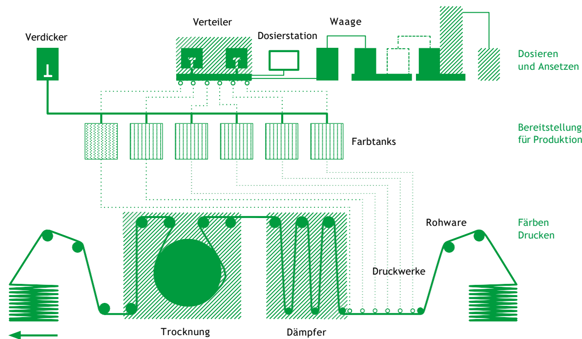
DIE FARBDOSIER- UND ANSATZSTATION
